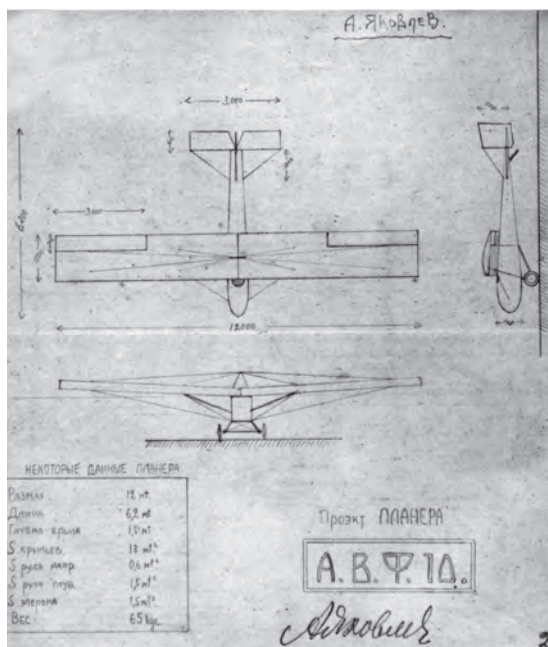
Чертеж планера АВФ-10, разработанного А.С. Яковлевым в Академии воздушного флота
