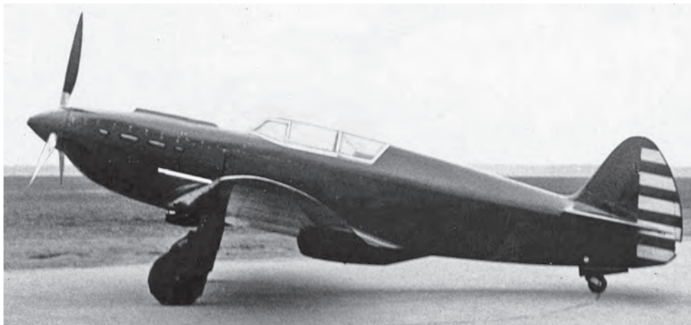
Опытный истребитель А.С. Яковлева И-26, поднявшийся в воздух 13 января 1940 г.
